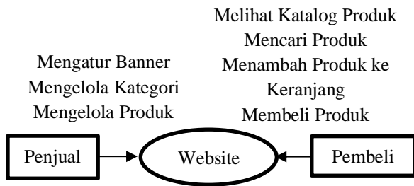
Gambar 4 Diagram konteks
